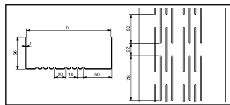
SKY Vnější stěnový vodící profil
